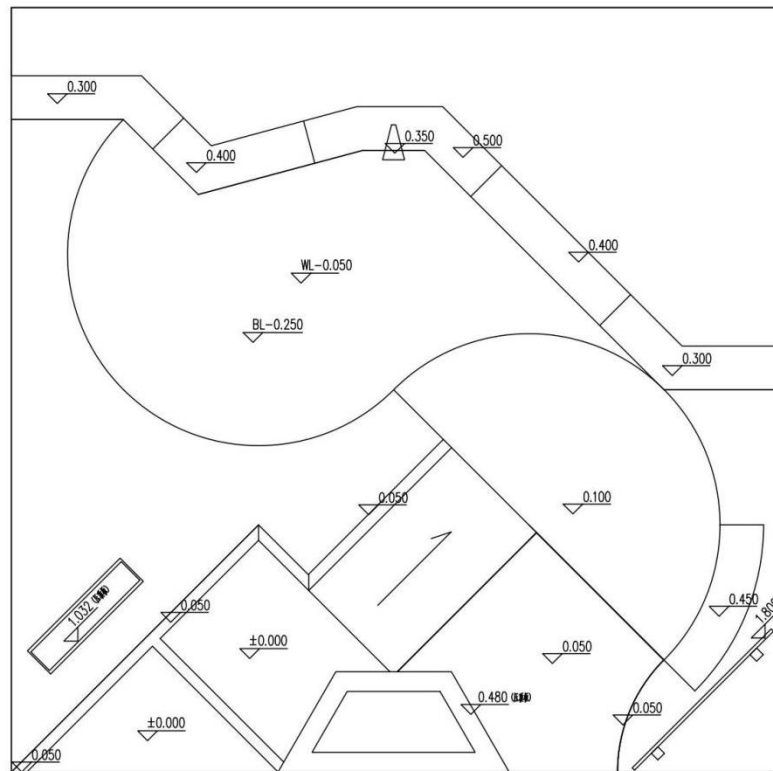
竖向标高图
